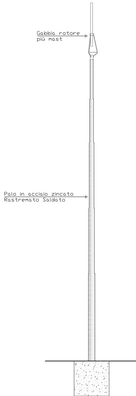
PROSPETTO / SEZIONE SUPPORTO ANTENNA
